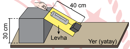
II. Düzenek
