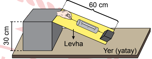
I. Düzenek
